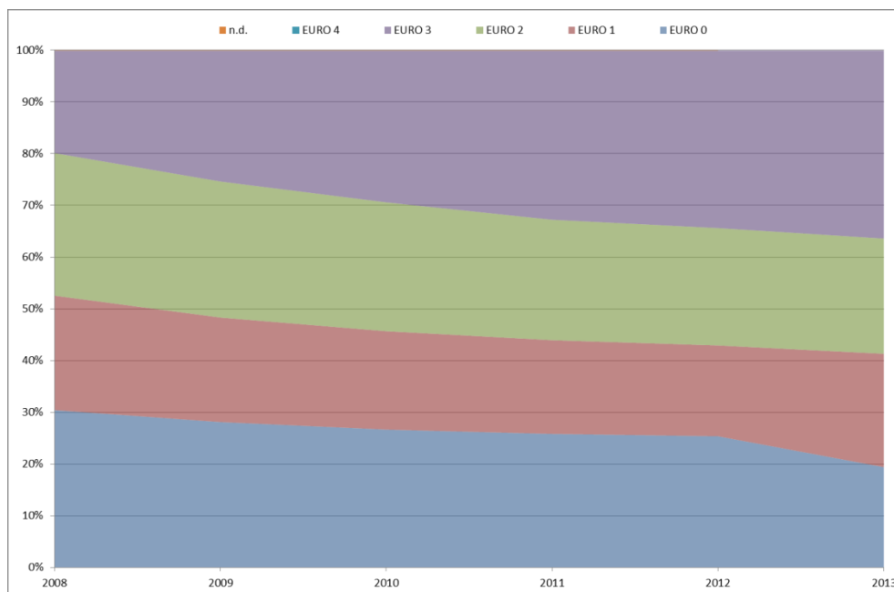
Grafico 14 – Motocicli circolanti per direttiva europea antinquinamento dal 2008 al 2013
