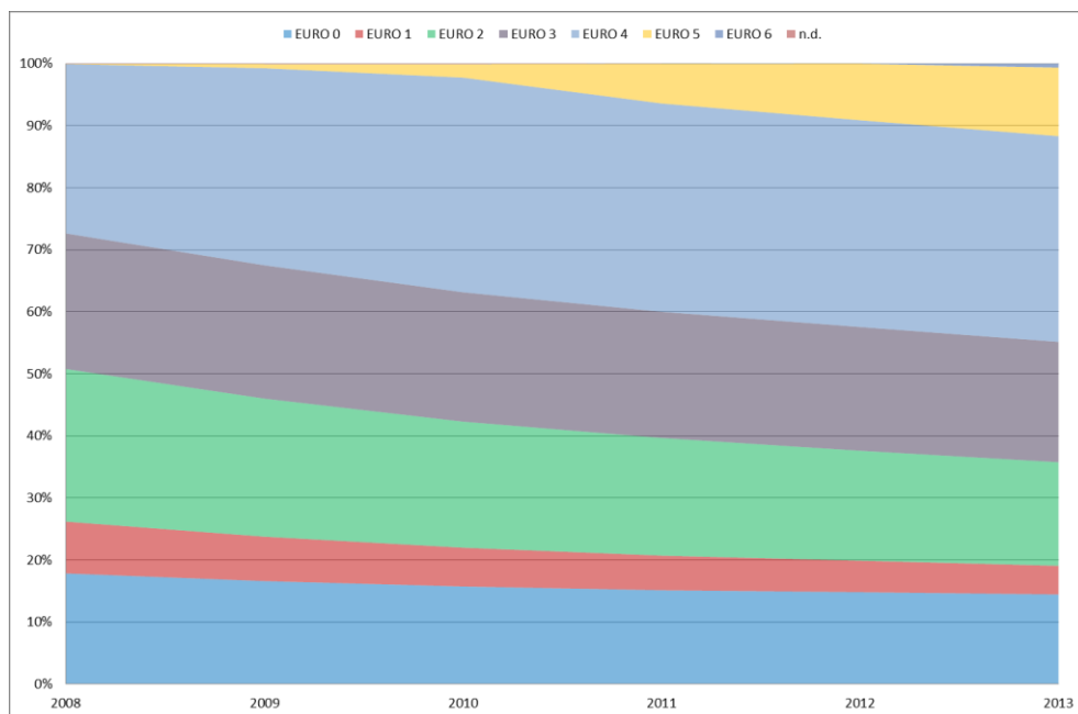
Grafico 12 – Autovetture circolanti per direttiva europea antinquinamento dal 2008 al 2013
