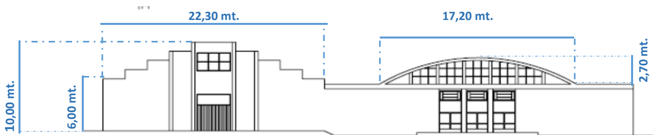
PROSPETTO PRINCIPALE
