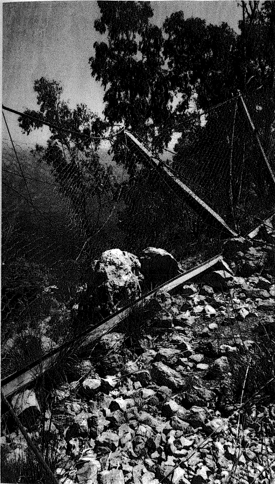
F.2 particolare massi imbrigliato dalla rete paramassi
