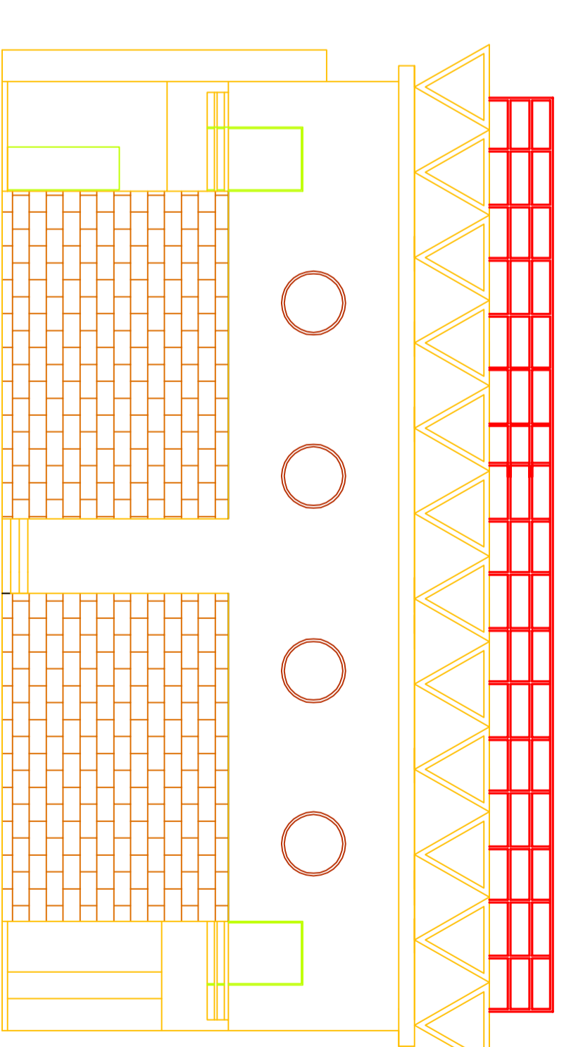
PROSPETTO NORD
