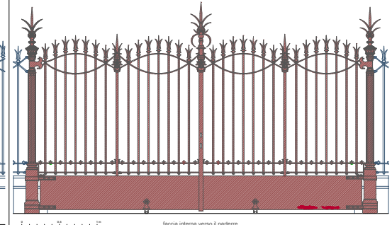
faccia interna verso il parterre
