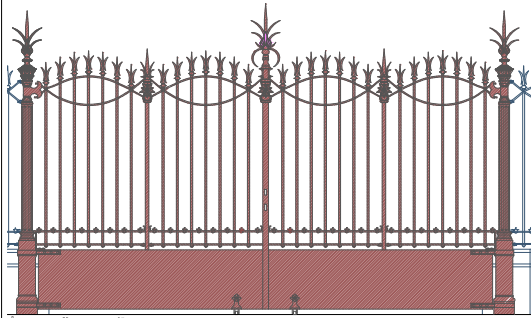
faccia interna verso il parterre
