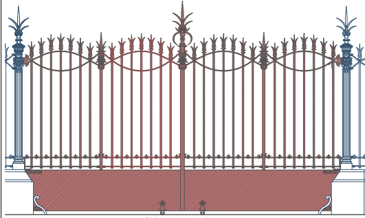
faccia esterna verso la piazza
