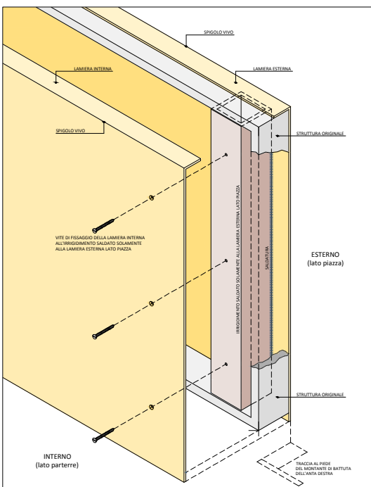
PARTICOLARE DELL'IRRIGIDIMENTO - Scala 1:2
