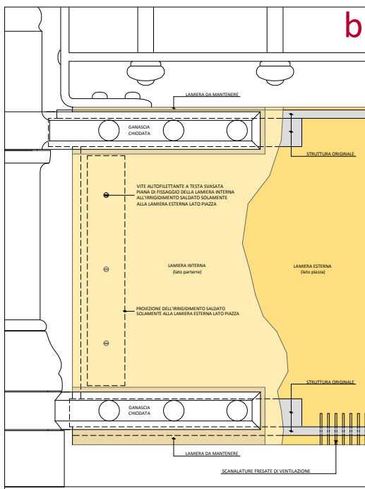
PARTICOLARE IN PROSSIMITÀ DELLE GANASCE CHIODATE - Scala 1:2
