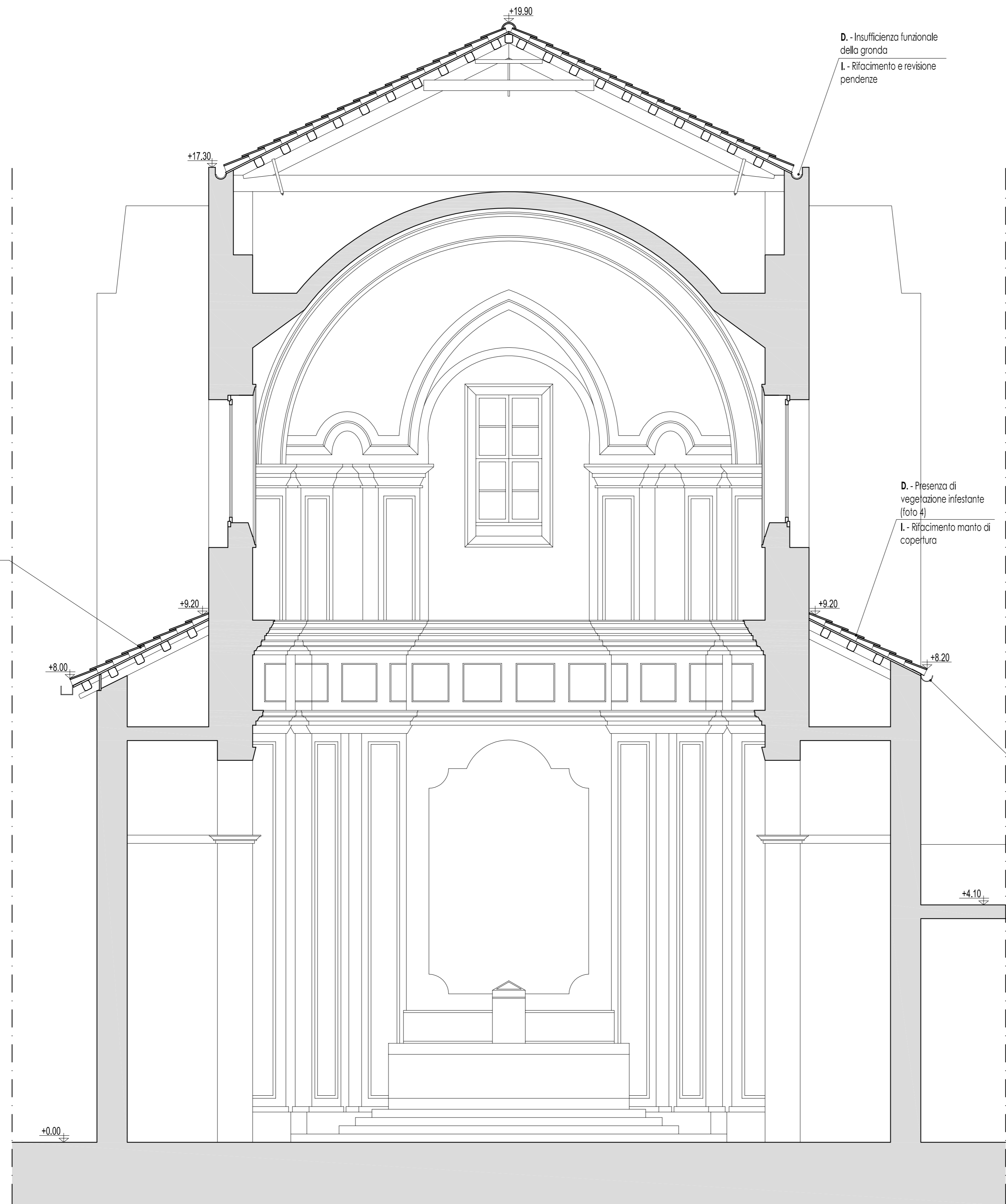
Sezione I-I scala 1:50
