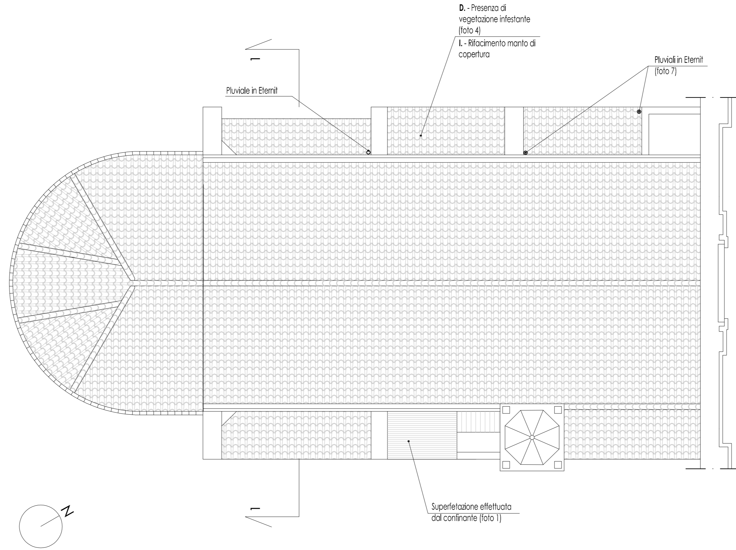
Pianta copertura scala 1:100
