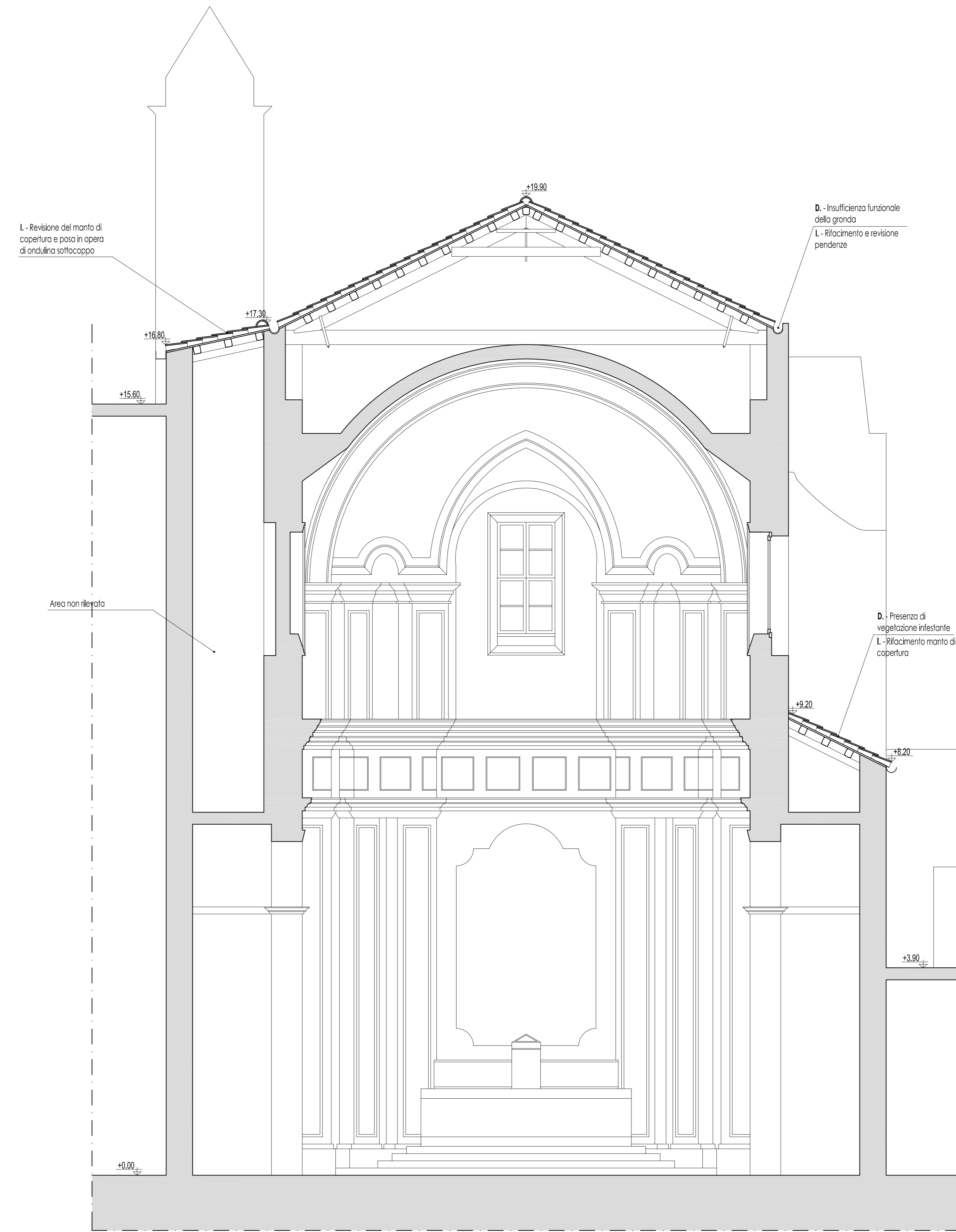
Sezione 3-3 scala 1:50
