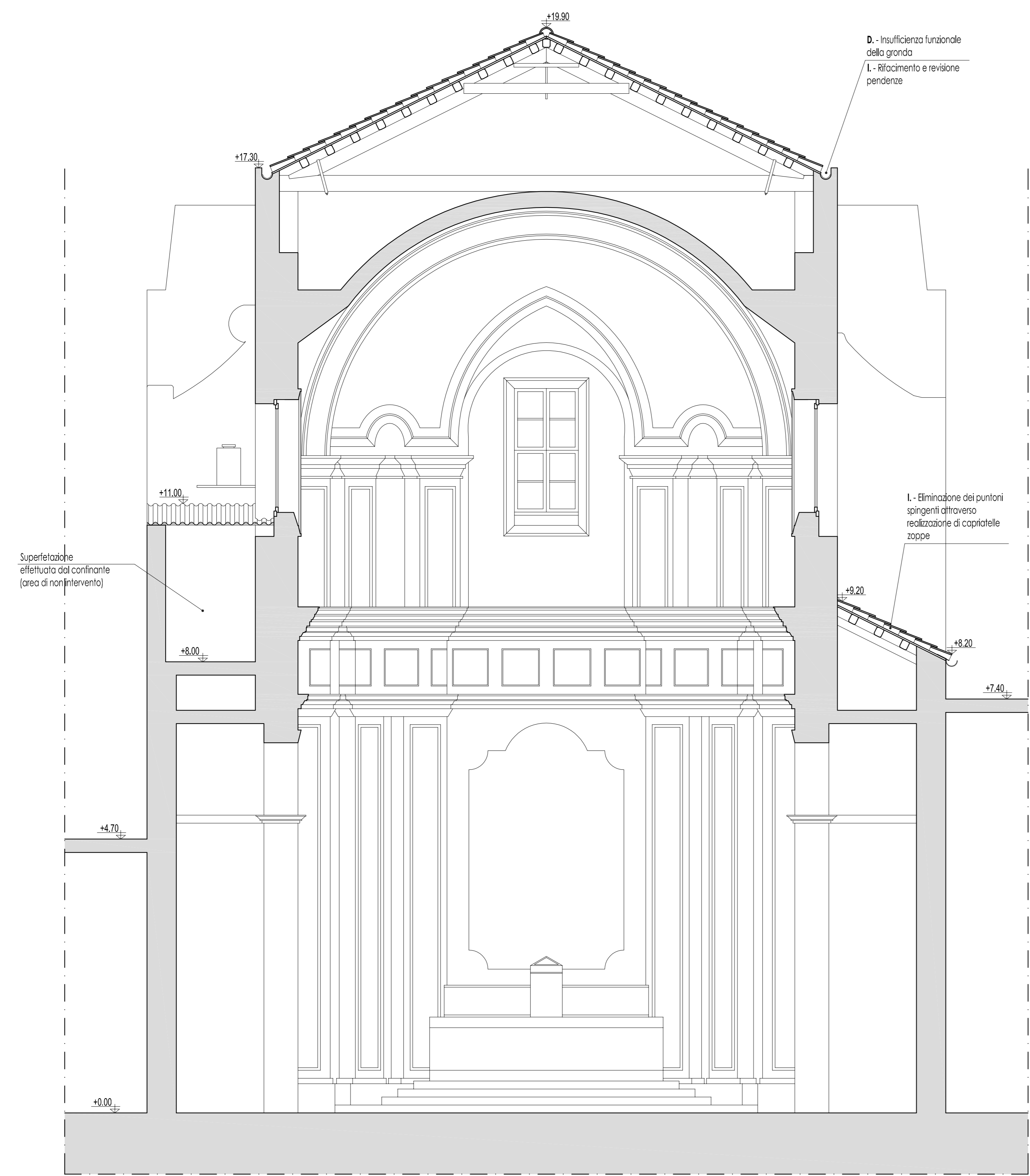
Sezione 2-2 scala 1:50
