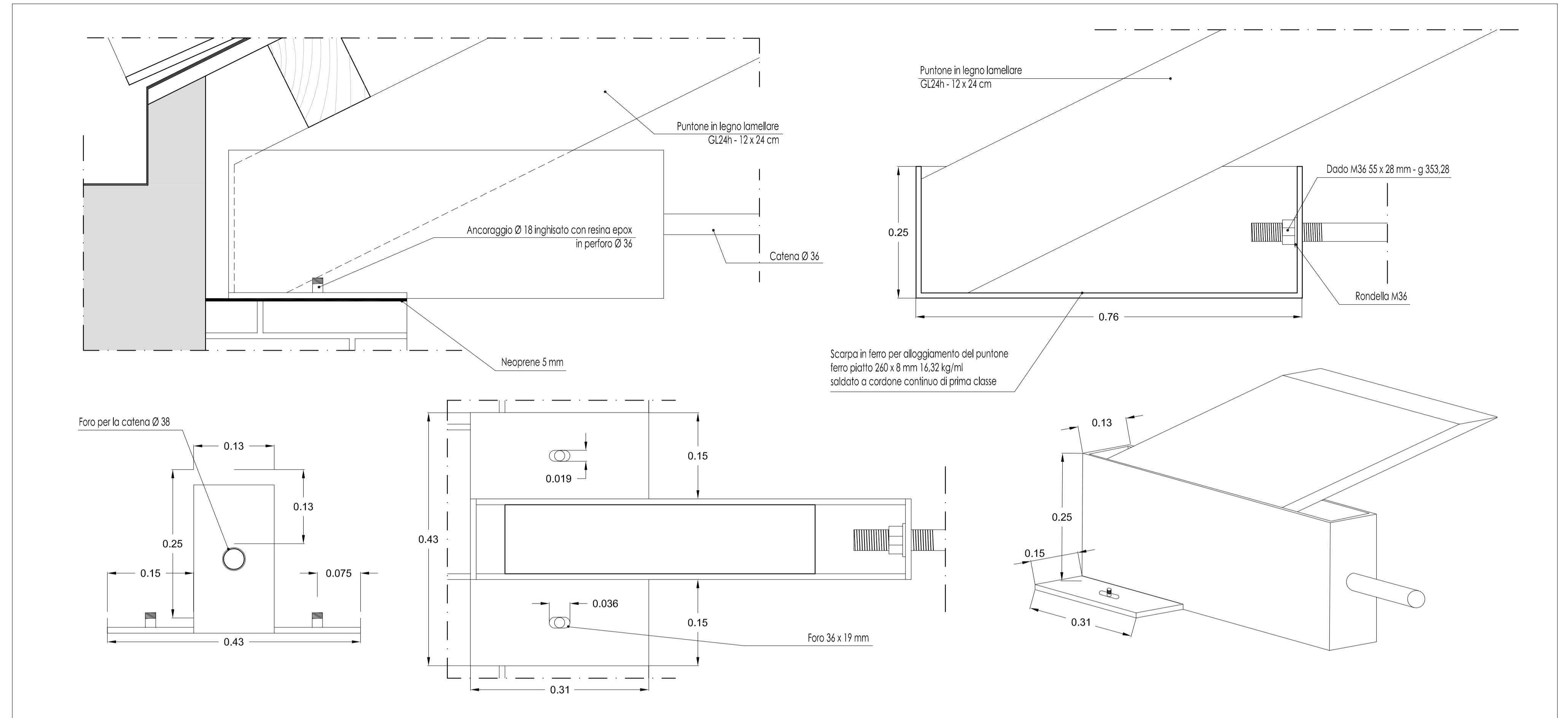
Particolare della scarpa scala 1:5
