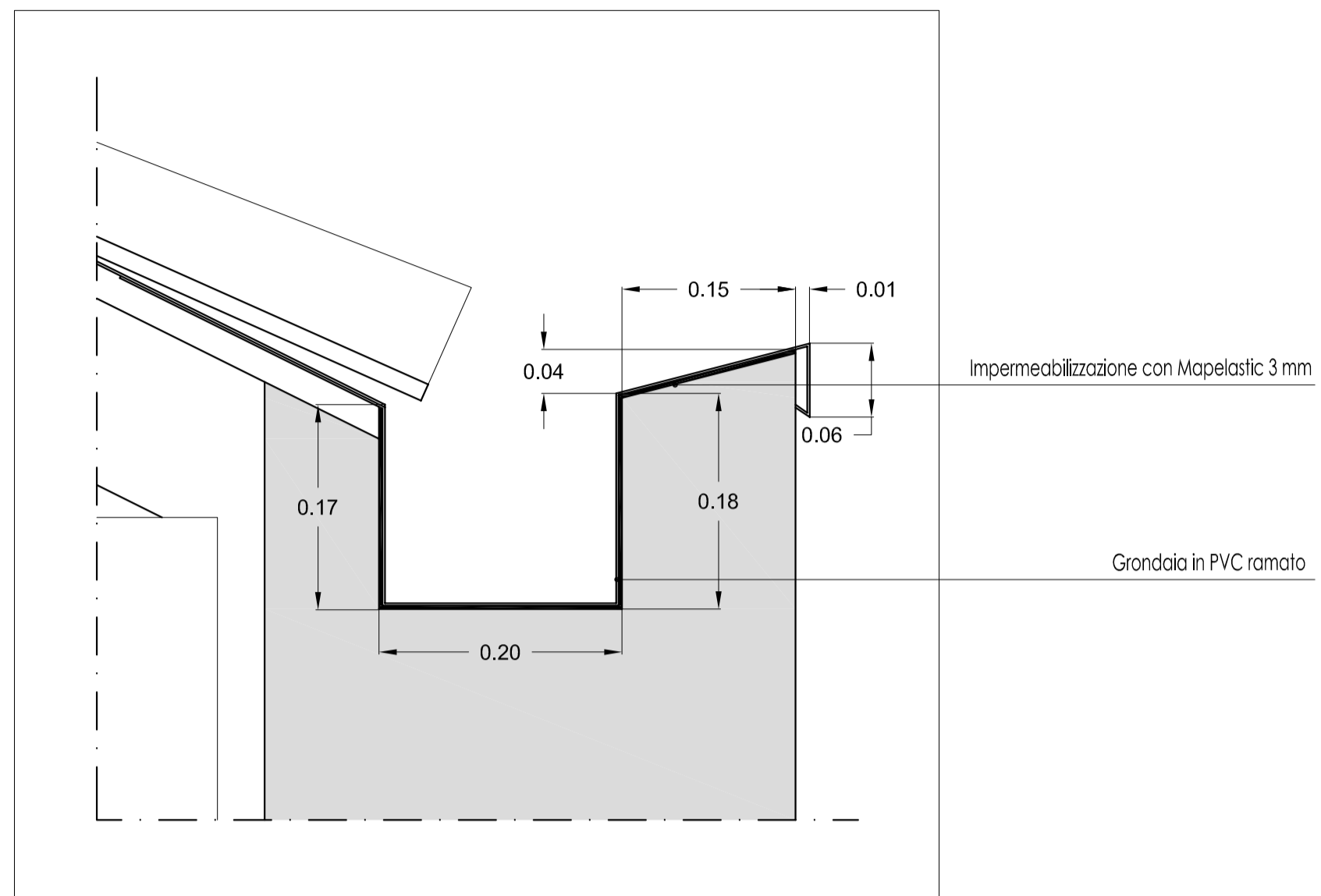
Particolare grondaia scala 1:5
