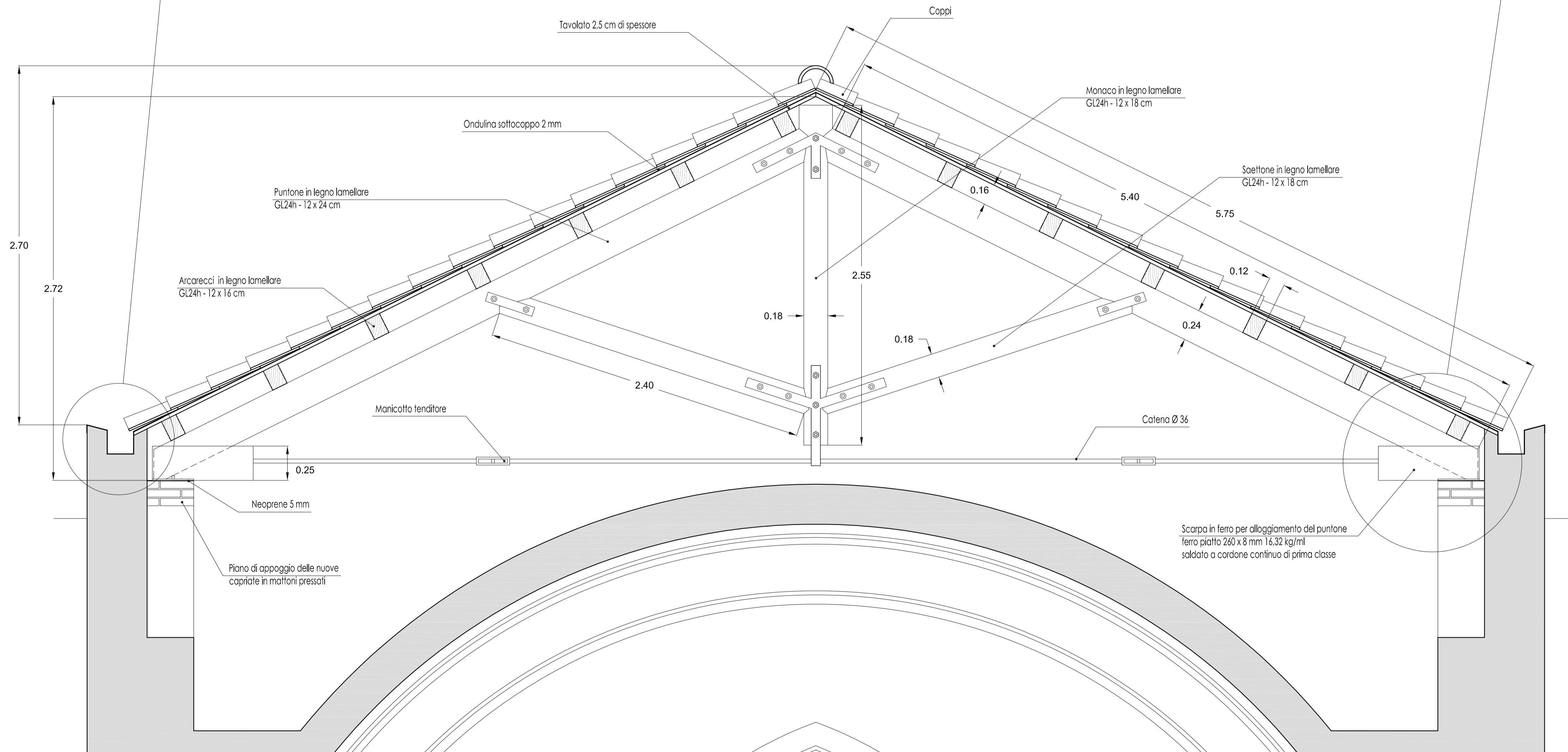
Capiata della navata scala 1:20
