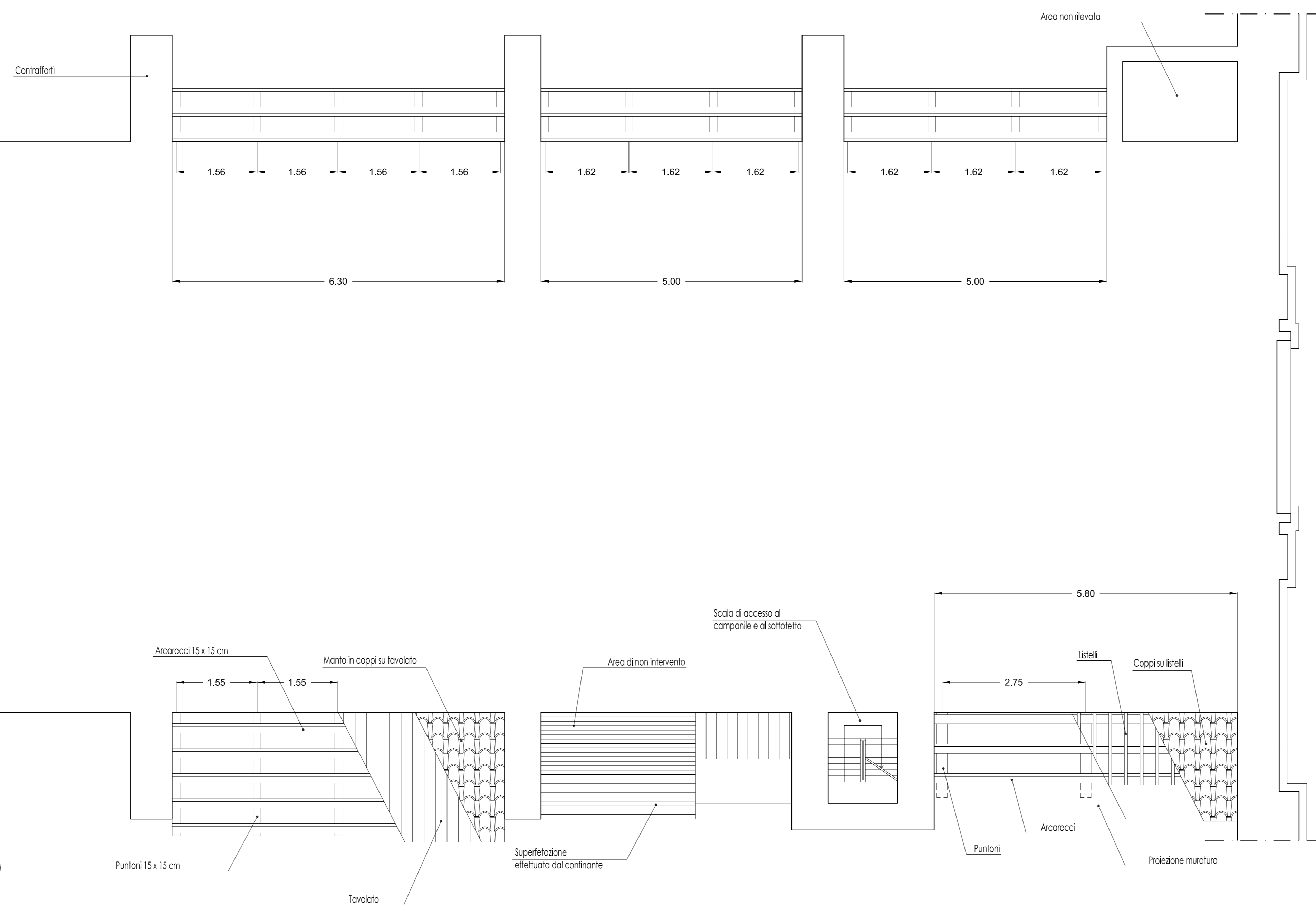
Sistema di copertura delle cappelle laterali scala 1:50
