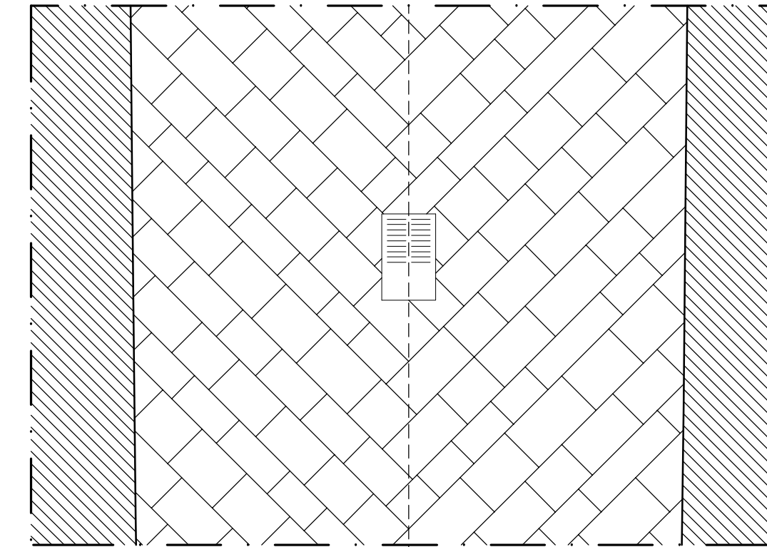
Sezione tipo 3 (vicolo Papireto)
