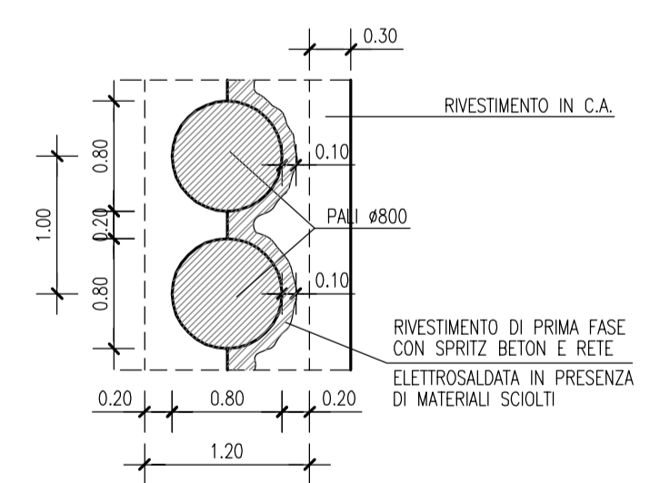
PARTICOLARE PARATIA DI PALI TRIVELLATI _ 1:50
