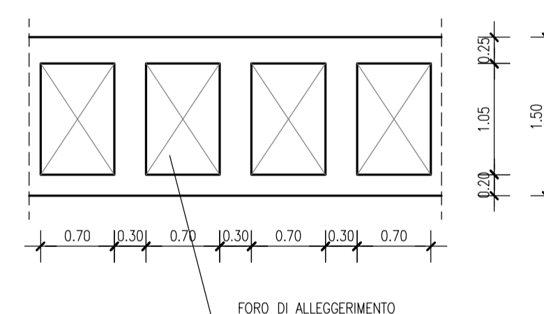
PARTICOLARE SOLAIO COPERTURA _ 1:50
