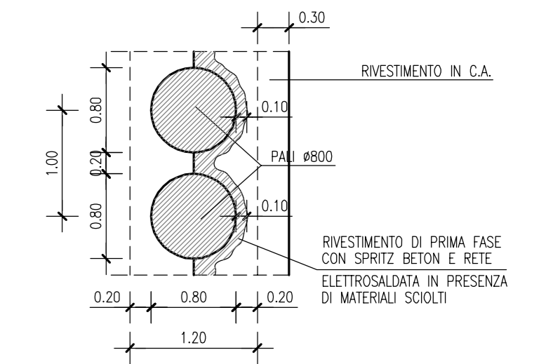
PARTICOLARE PARATIA DI PALI TRIVELLATI _ 1:50
