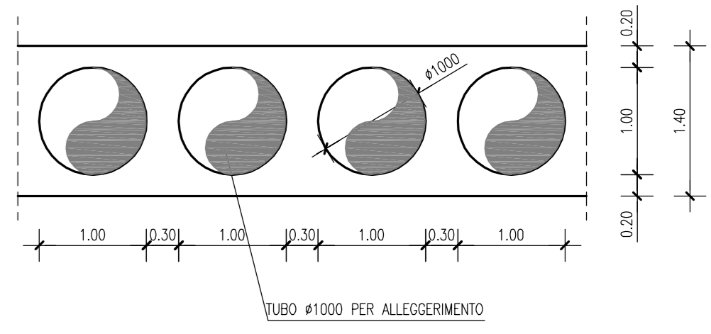
PARTICOLARE SOLAIO PIANO INTERMEDIO _ 1:50
