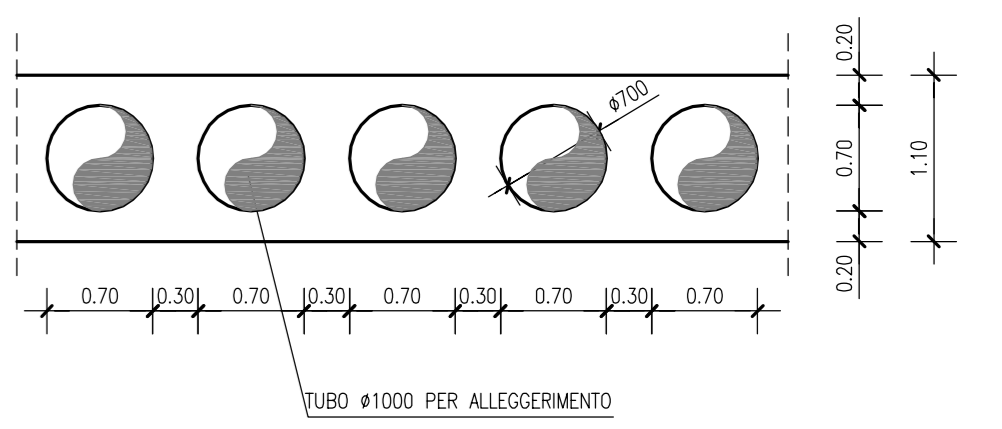
PARTICOLARE SOLAIO PIANO INTERMEDIO _ 1:50
