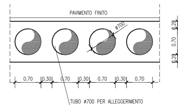
PARTICOLARE SOLAIO ATRIO _ 1:50
