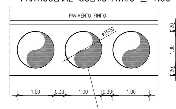
PARTICOLARE SOLAIO ATRIO _ 1:50
