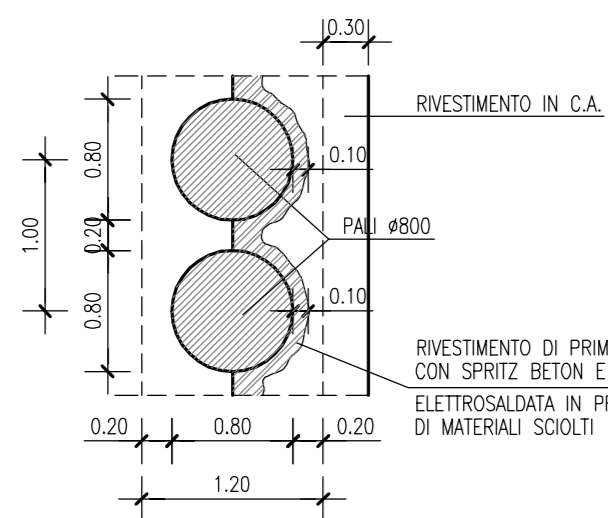
PARTICOLARE PARATIA DI PALI TRIVELLATI _ 1:50
