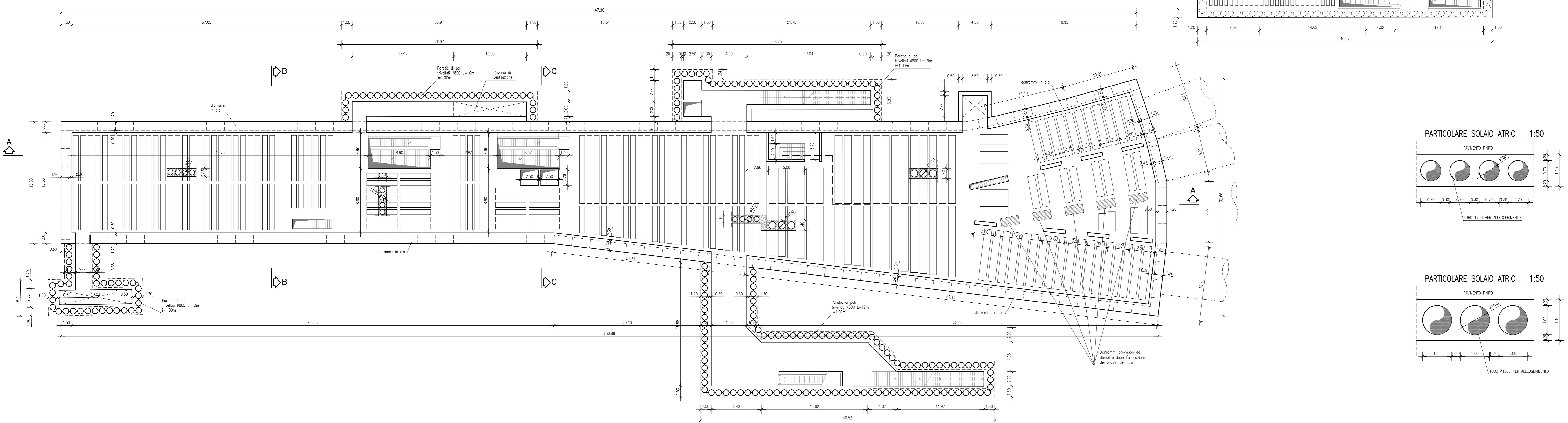
STAZIONE ARCHIMEDE-BIVIO / PIANO ATRIO QUOTA (-7.30;-8.00) _ 1:200
