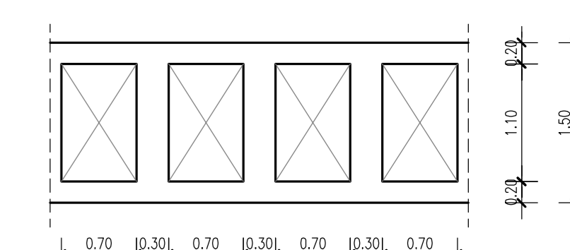
PARTICOLARE SOLAI COPERTURA _ 1:50
