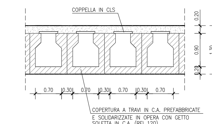
PARTICOLARE TRATTO DI COPERTURA _ 1:50 IN ELEMENTI PREFABBRICATI IN C.A.
