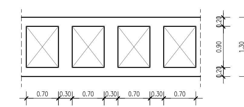
PARTICOLARE SOLAI COPERTURA _ 1:50
