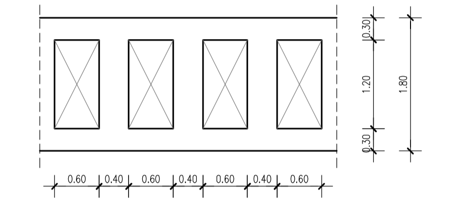
PARTICOLARE SOLAIO PIANI INTERMEDI _ 1:50
