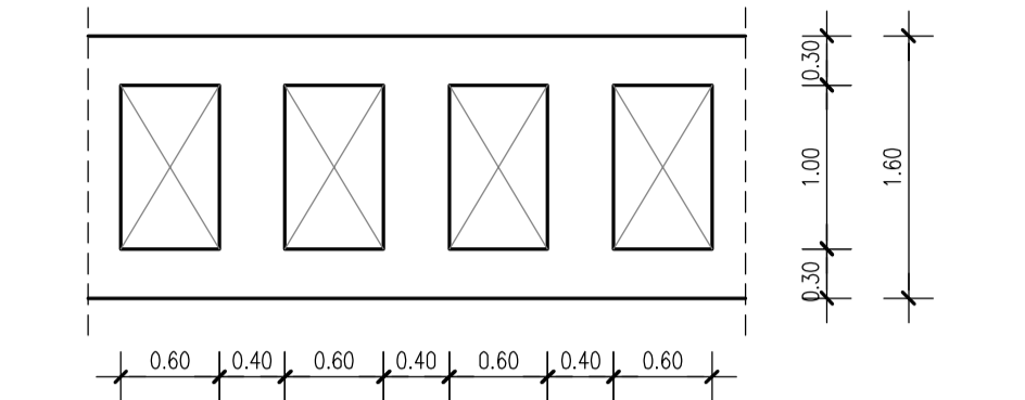
PARTICOLARE SOLAIO PIANI INTERMEDI _ 1:50
