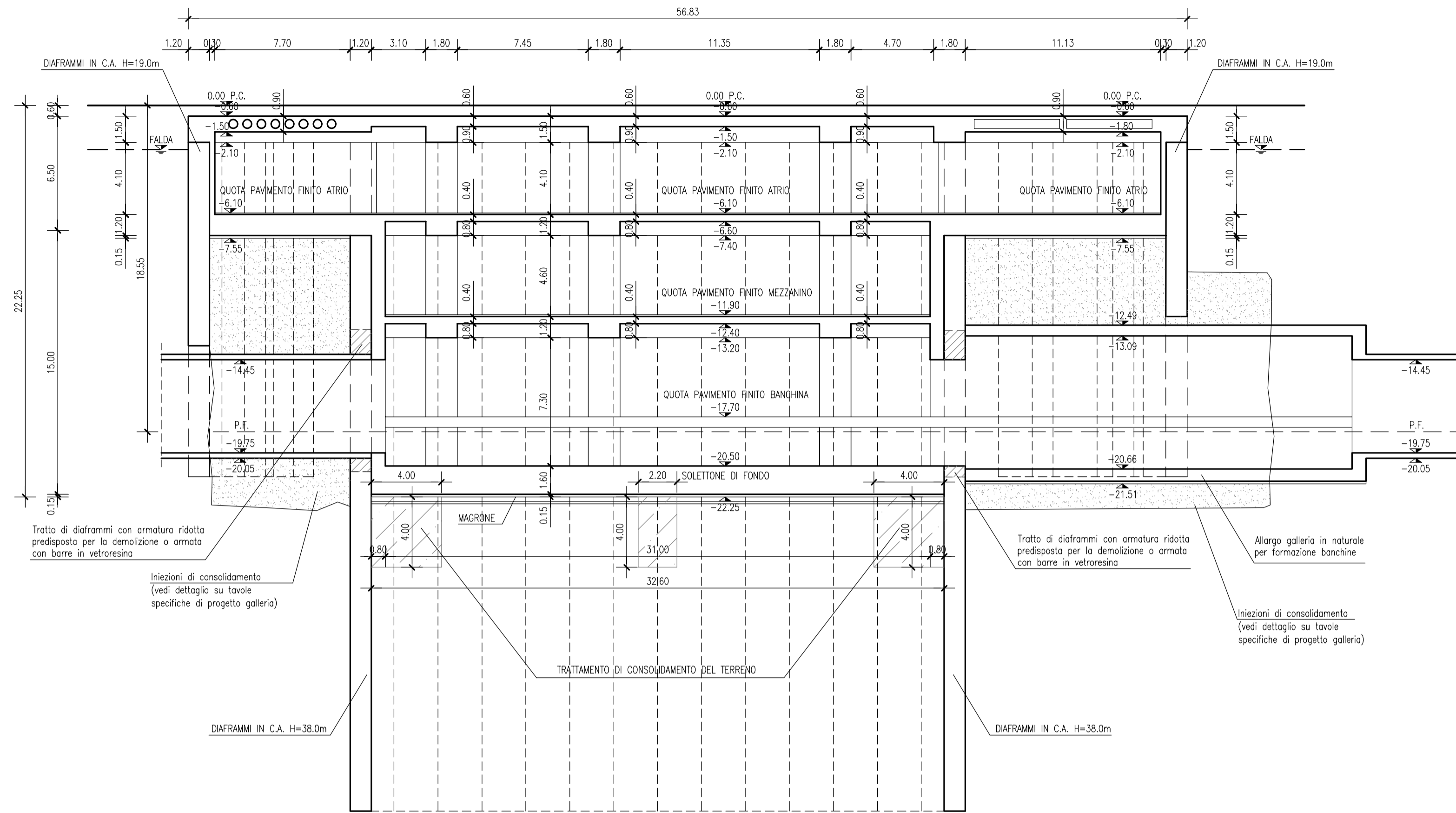
STAZIONE BORSA / SEZIONE B-B _ 1:200
