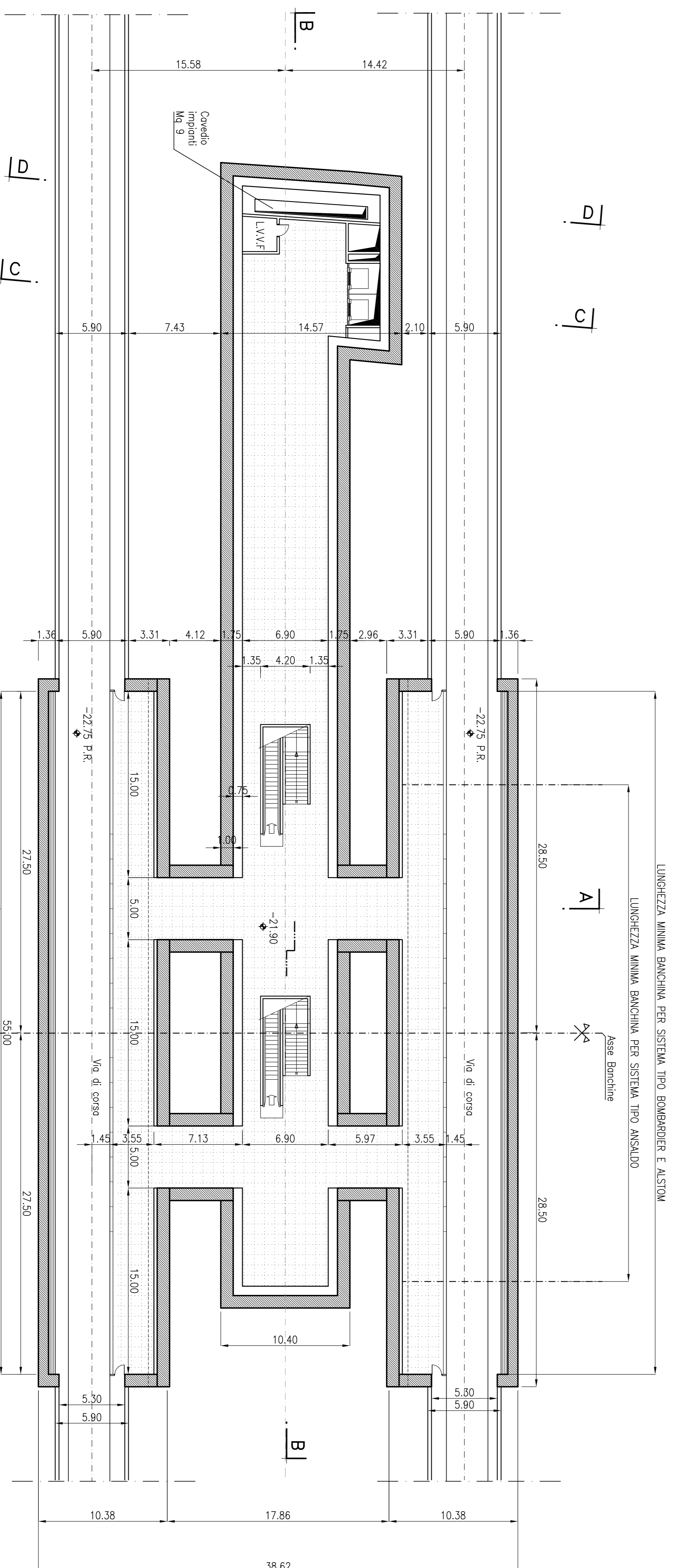
PIANO A QUOTA (-21.90)
