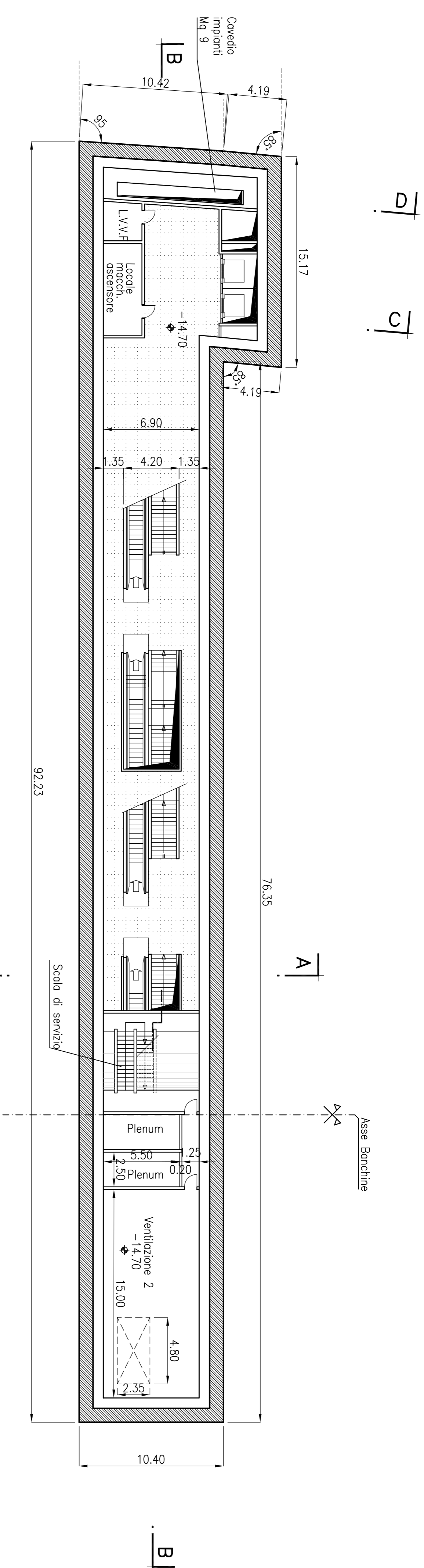
PIANO A QUOTA (-14.70)
