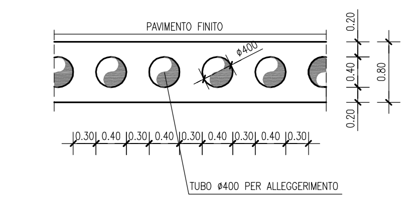
PARTICOLARE TRAVE ZONA ACCESSI _ 1:50
