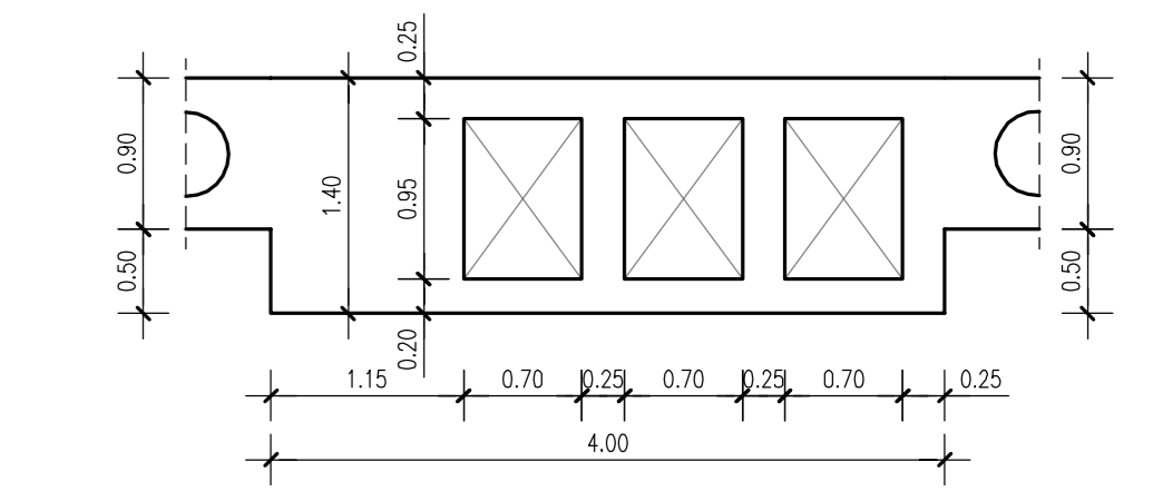
PARTICOLARE TRAVE ZONA ACCESSI _ 1:50
