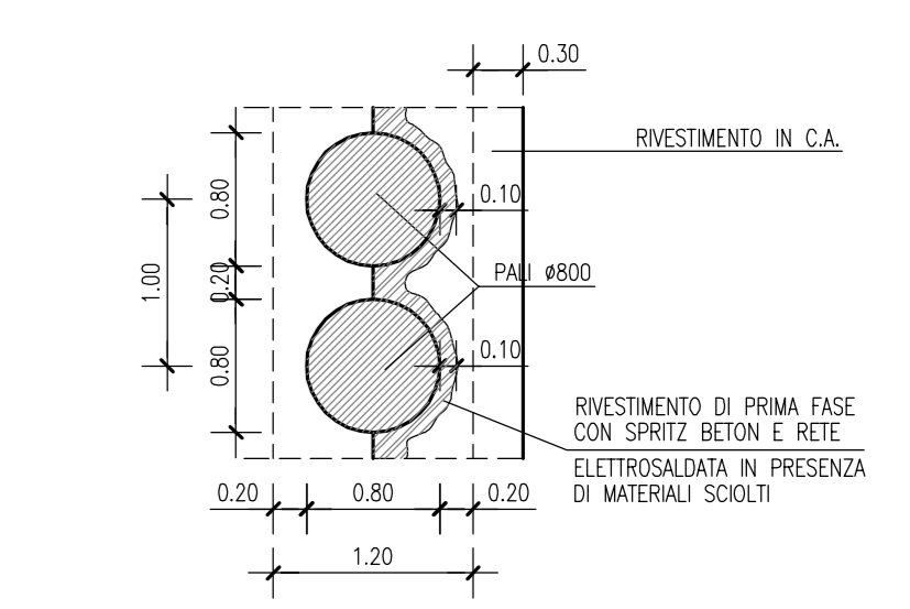
PARTICOLARE PARATA DI PALI TRIVELLATI _ 1:50
