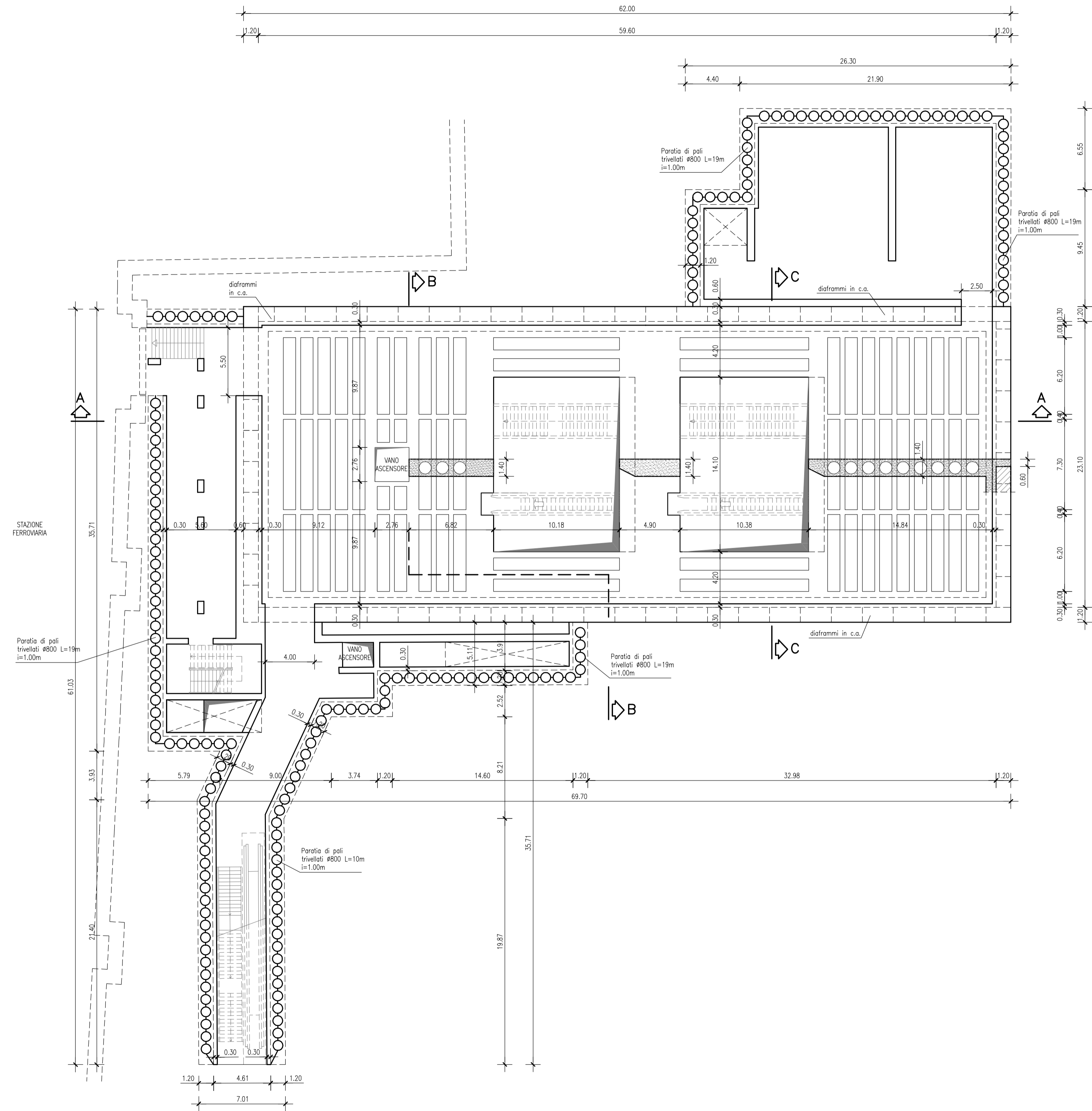
PIANTA PIANO ATRIO QUOTA (-7.10) _ 1:200
