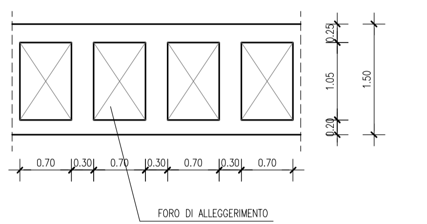
PARTICOLARE SOLAIO COPERTURA _ 1:50
