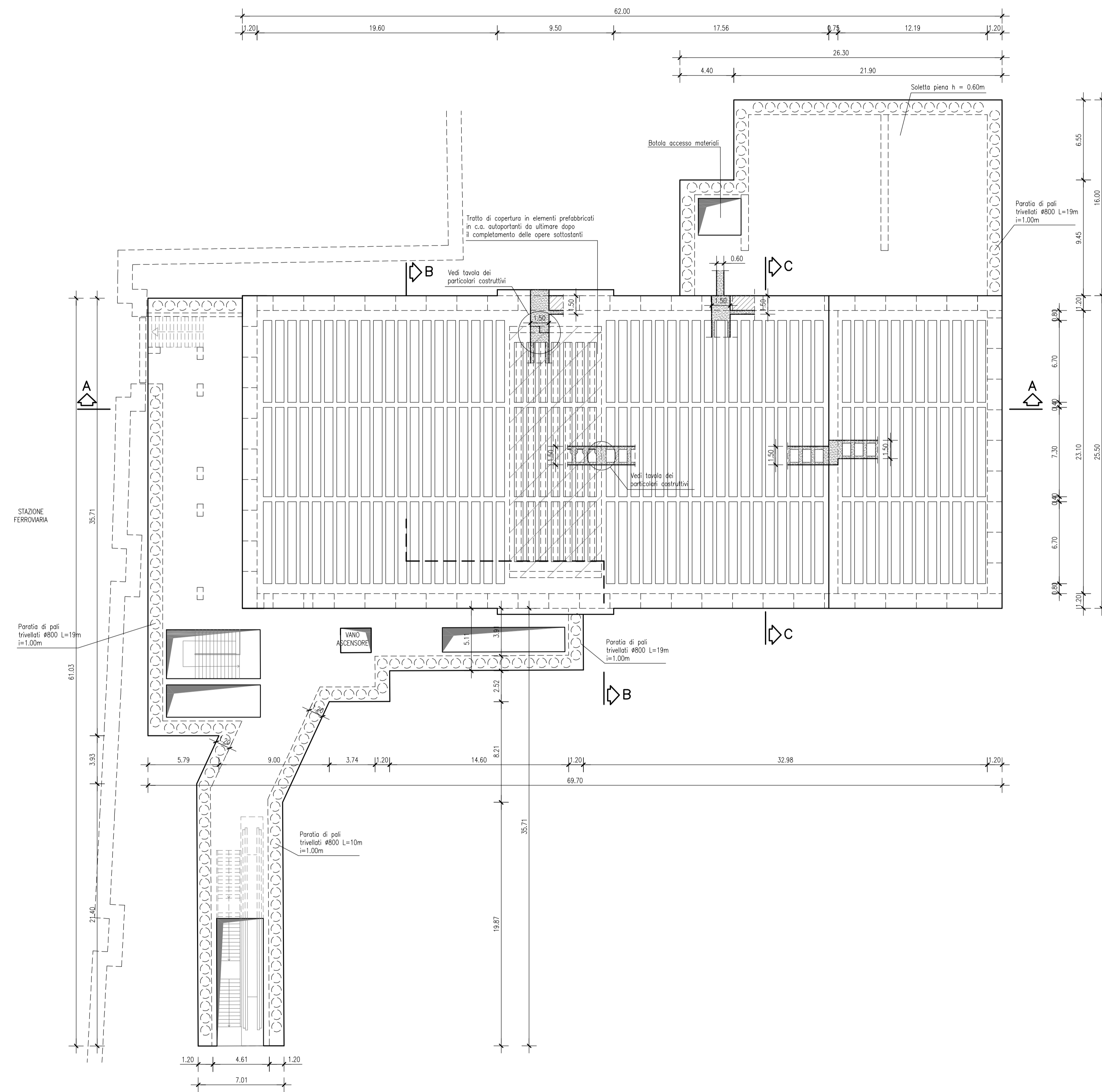
PIANTA SOLETTONE DI COPERTURA QUOTA (-1.10;-1.60;-2.00) _ 1:200
