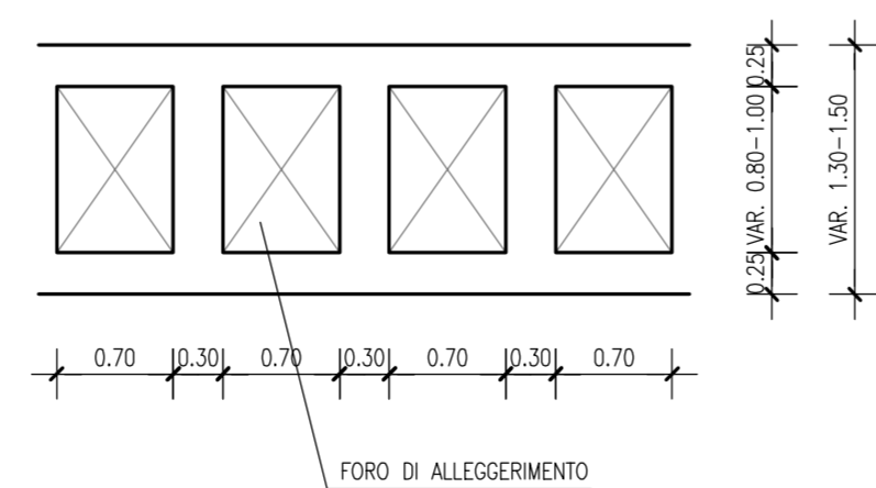
PARTICOLARE SOLAIO COPERTURA _ 1:50
