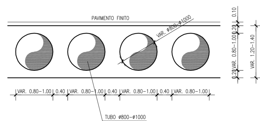
PARTICOLARE SOLAIO COPERTURA _ 1:50
