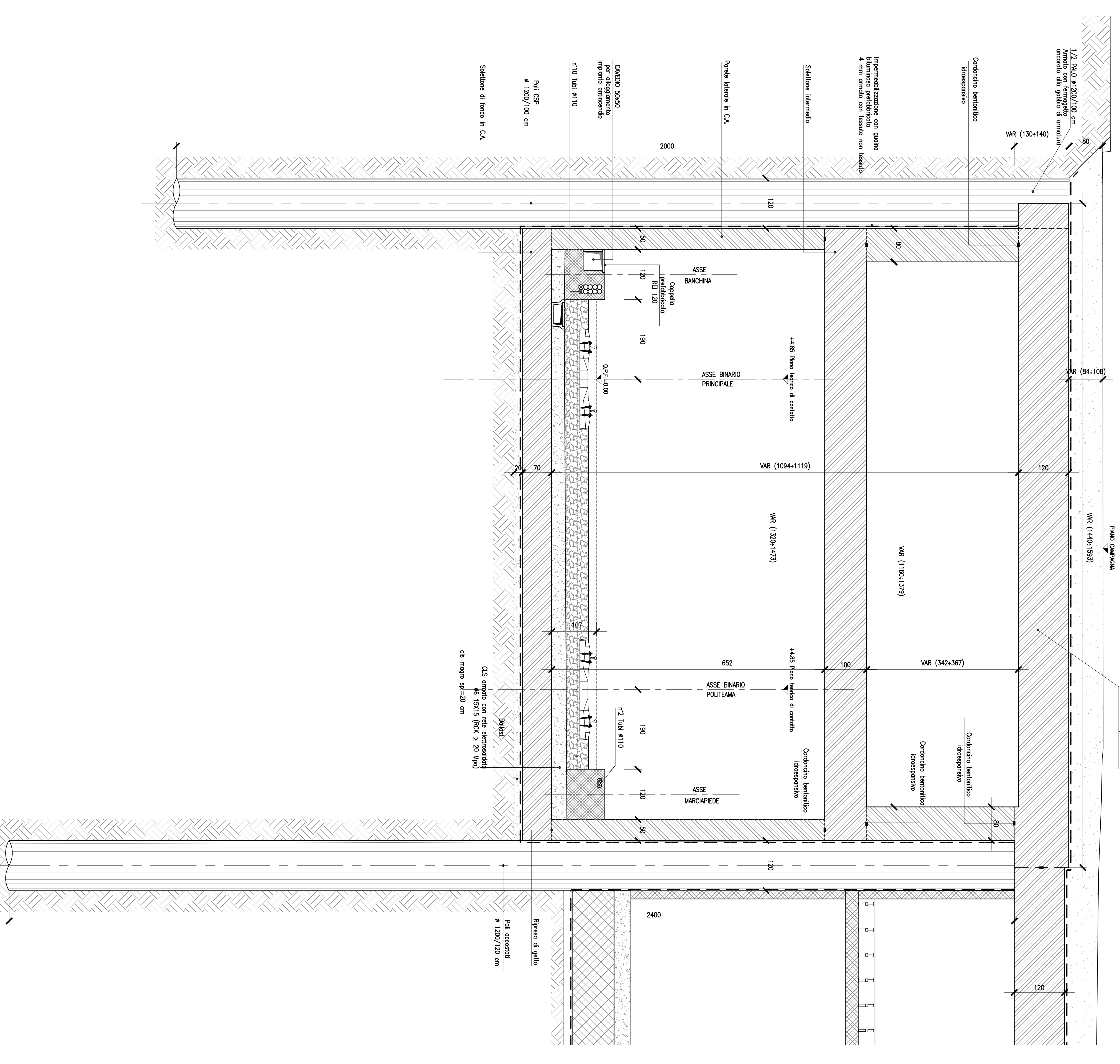
SEZIONE TIPO "3"-Scida 1:50
