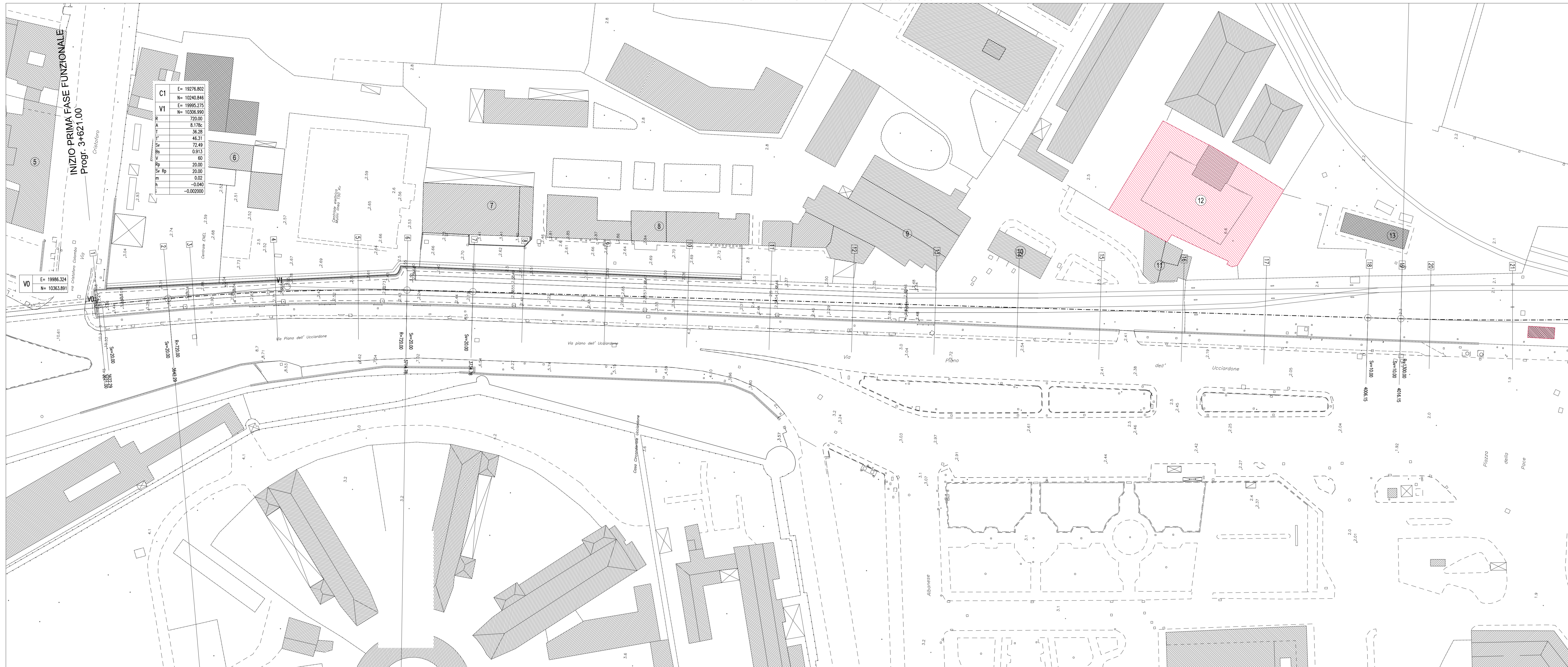
PLANIMETRIA DI TRACCIAMENTO Tav. 2 di 4 - Scala 1:500 -
