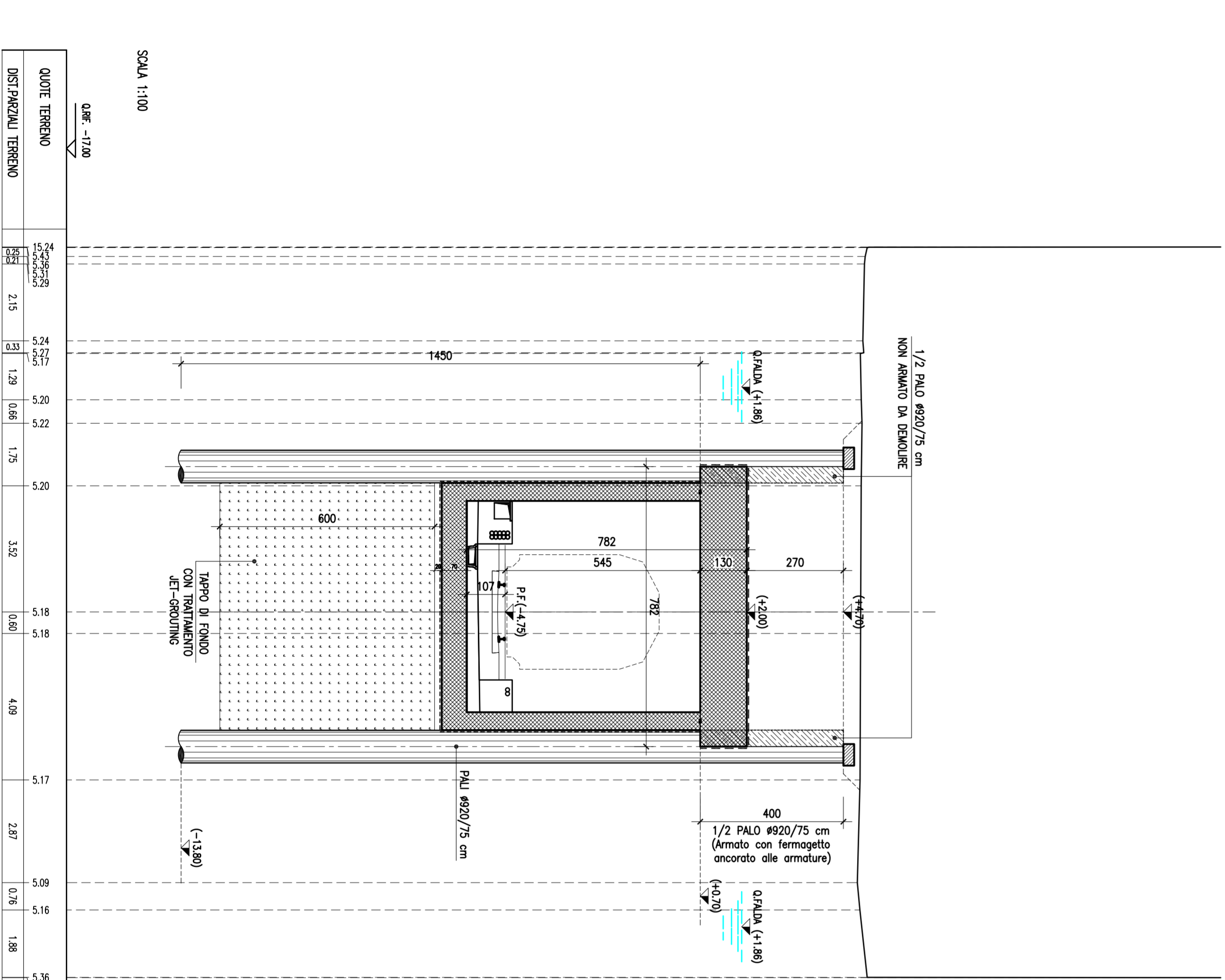
SEZIONE N. : 47 Q. PROGETTO : -4/416 DATA: 03/08
