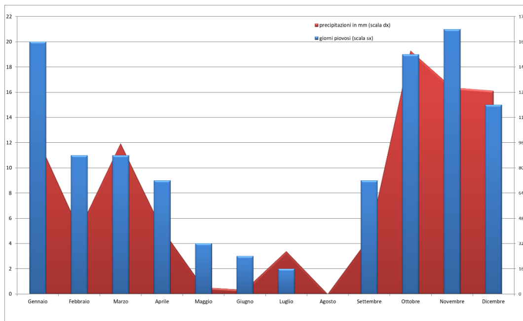
Grafico 2.4: Precipitazioni (in mm) e numero di giorni piovosi per mese nel 2021
