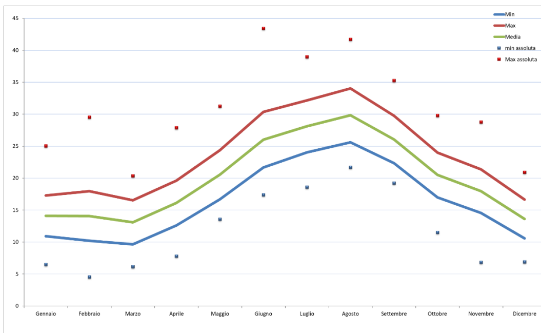
Grafico 2.3: Temperatura minima, media e massima nel 2021
