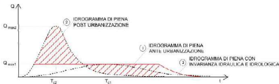
Fig. 2 – Rappresentazione delle portate ANTE e POST urbanizzazione tenendo conto dell'invarianza idraulica
