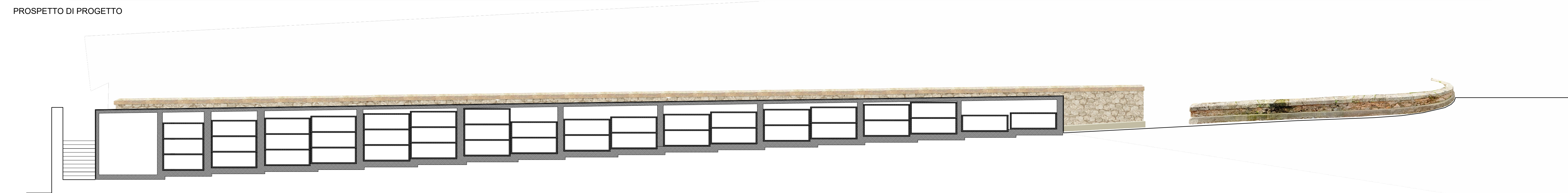
SEZIONE A - A' DI PROGETTO
