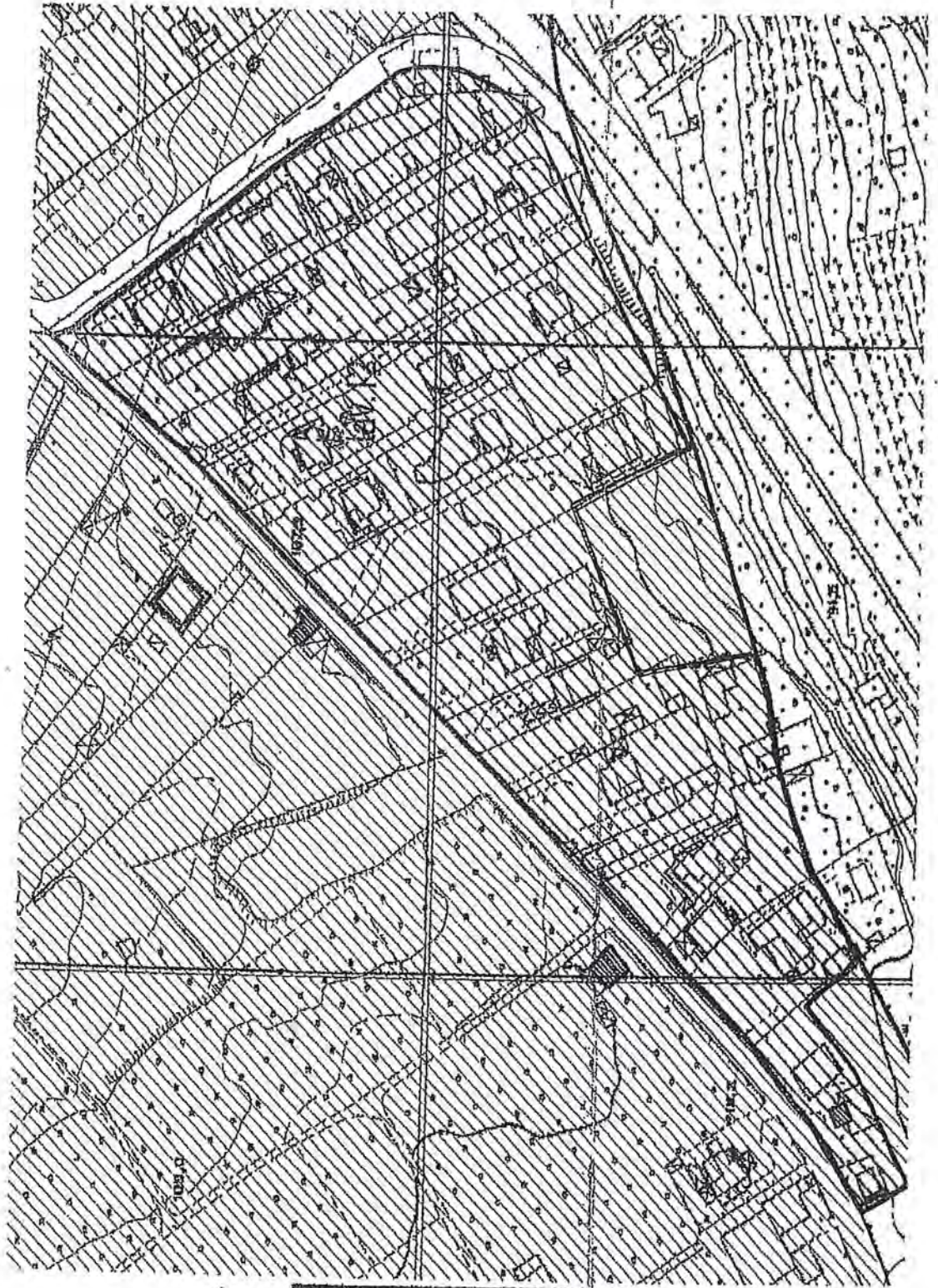
5 TAV. 12 - SCALA 1:2000
