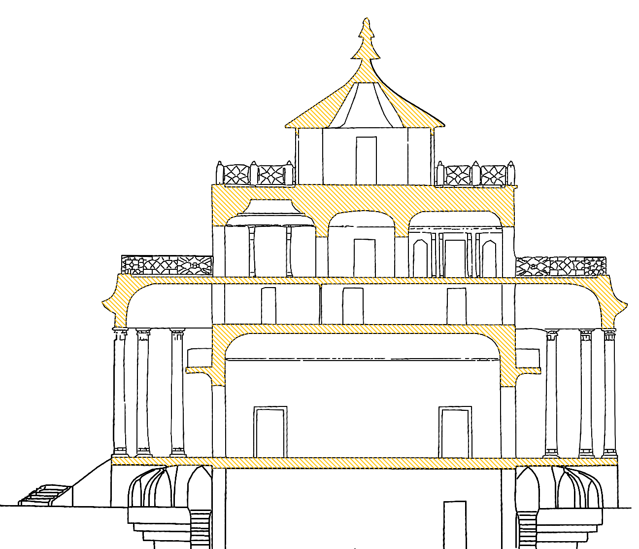
Sezione Casina cinese
