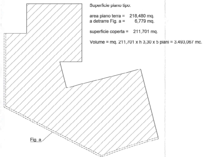
SAGOMA PIANO TIPO (Piani 1-5)
